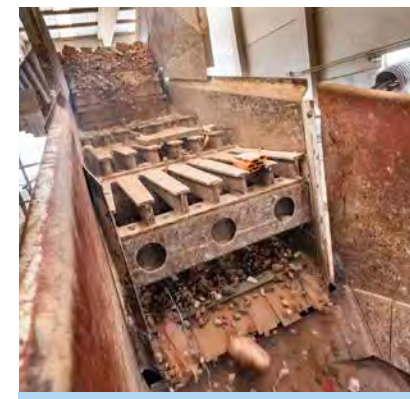
Vorabscheider mit Unwuchterreger zur Aufbereitung von Bauschutt Grizzly feeder with unbalanced exciter for processing construction waste
