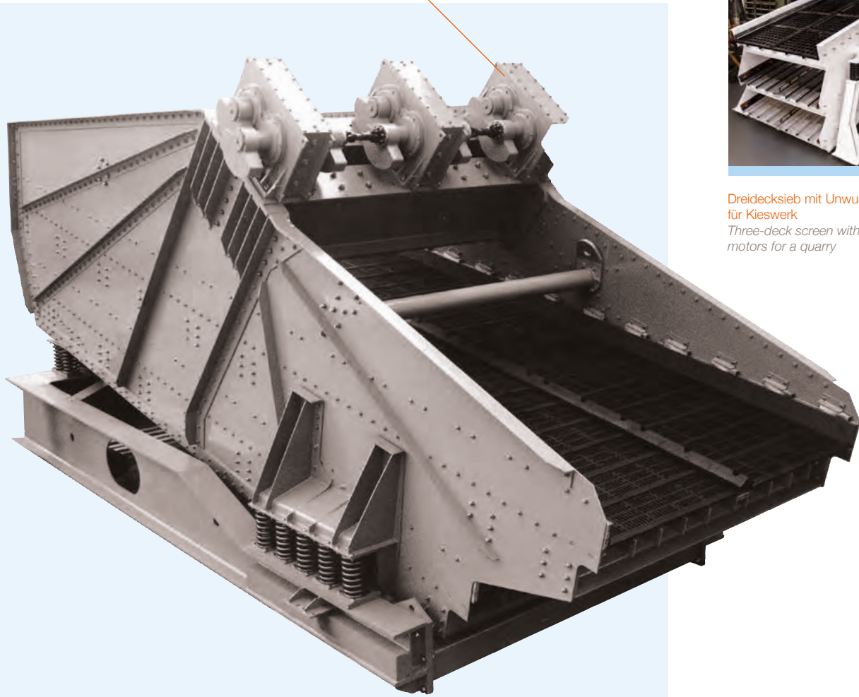
Doppeldeck-Linearschwingsieb für eine Schiffsbeladeanlage Double-deck vibratory screen for a ship loading plant
