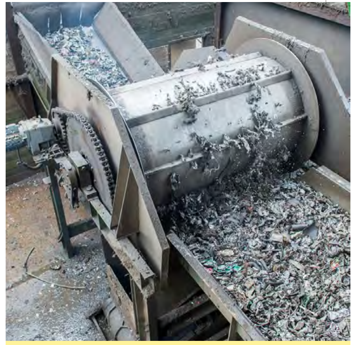
Förderrinne und Elektromagnettrummer in Schredderanlage Feeder and electromagnetic drum separator in a shredder plant
