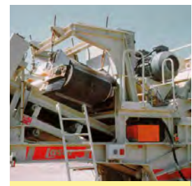
Diverse Überbandmagnetscheider für Fremdeisenentfernung Various magnetic overband separators for tramp iron removal
